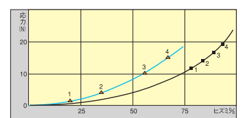
グラフ2 荷重一押込曲線(グラフ曲線上の数字1~4は、クッション中央下の圧力を示し、単位はkPa(1kPa=52mmHg))
